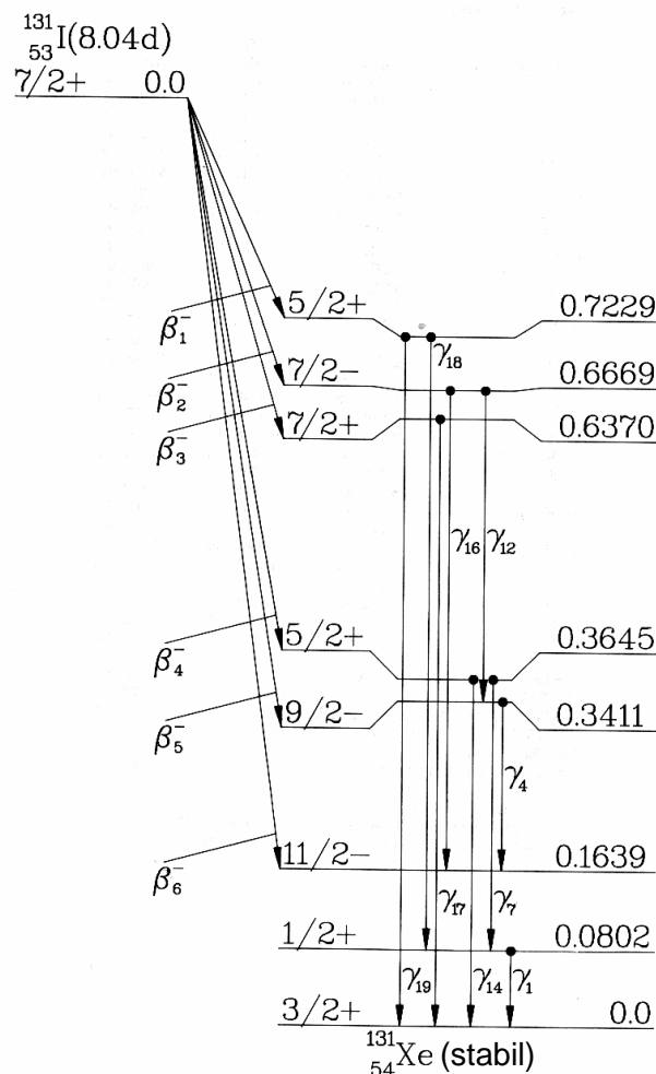
Schema de dezintegrare a ^{131}\text{I}
