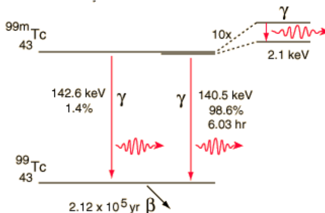
Schema de dezintegrare a ^{99m}\text{Tc}
